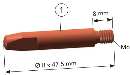
Type 3-2-__ /47.5
