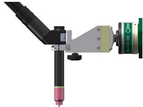
Adjusting gauge DIX EL 400 (optional)
