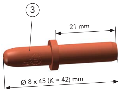
Type 3-2-__ SA(K)
